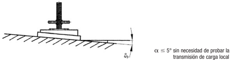
Figura 3-1 Ejemplo de una base distribuidora de la carga
