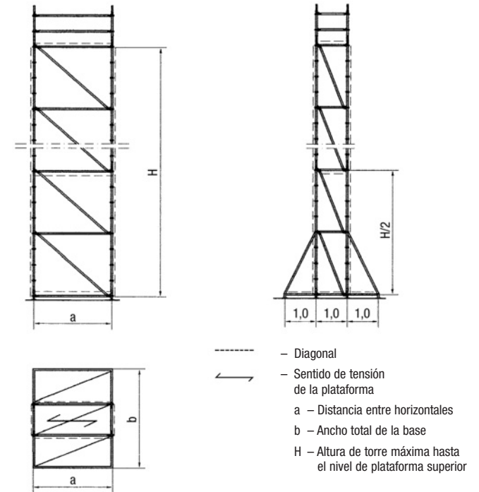
Barra para apoyar la plataforma según tabla de carga para barras horizontales
