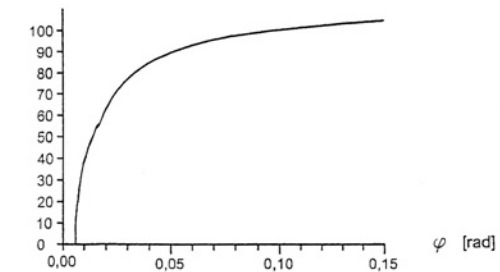
Figura 1: Rigidez de muelle giratorio media
