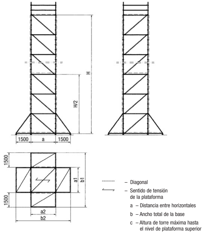
Barra para apoyar la plataforma según tabla de carga para barras horizontales
