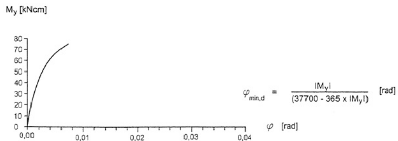
Figura 6: Rigidez de muelle giratorio máxima
