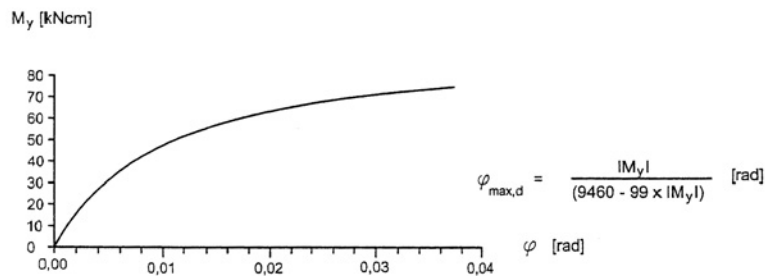
Figura 5: Rigidez de muelle giratorio mínima
