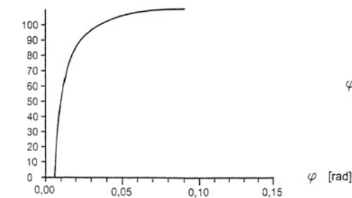
Figura 3: Rigidez de muelle giratorio máxima
